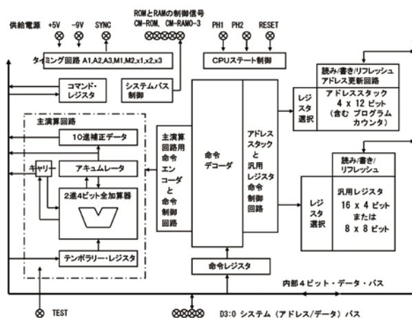
4004CPU ブロック図
