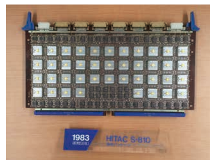
HITAC S-810 論理パッケージ
